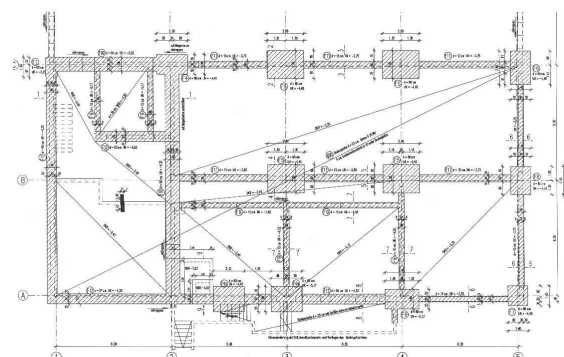
Grundriss Fundamente
