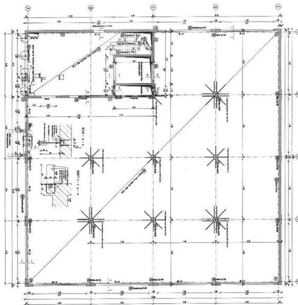
Grundriss Erdgeschoss
