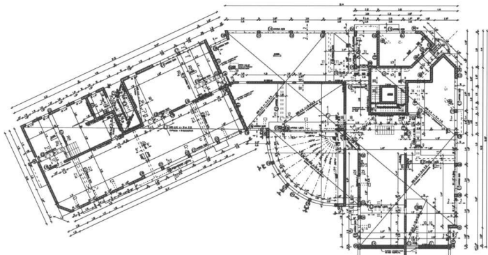
Grundriss Erdgeschoss Haus 3 und 4
