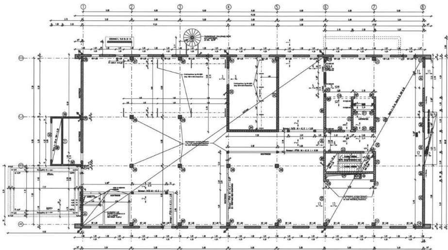
Grundriss Erdgeschoss
