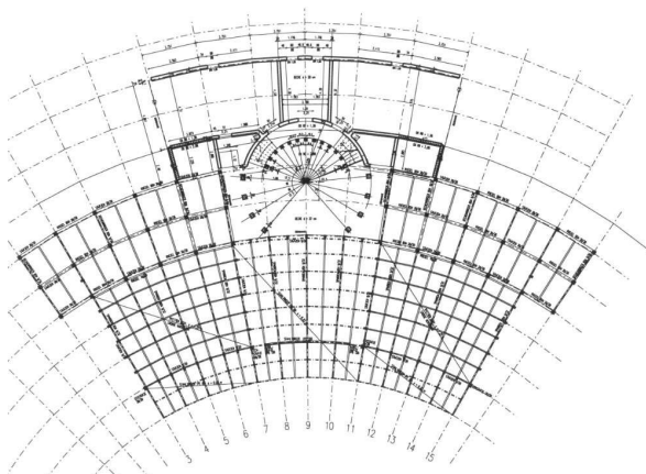
Holzbauplan Erdgeschoss
