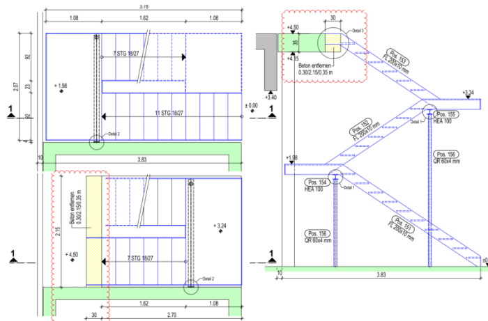
Grundriss und Schnitt Stahlterppe
