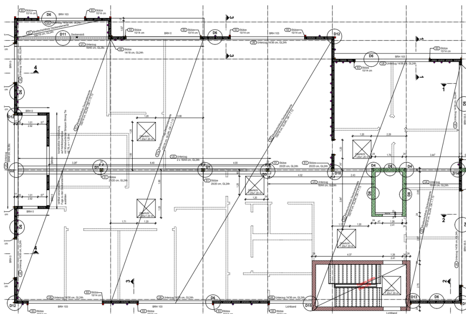
Grundriss Obergeschoss Aufstockung
