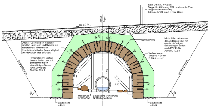
Querschnitt Gewölbebrücke
