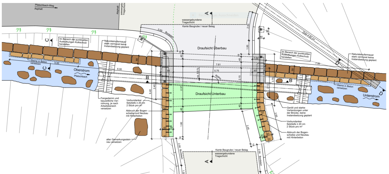
Grundriss Brücke mit bestehender Natursteinmauer
