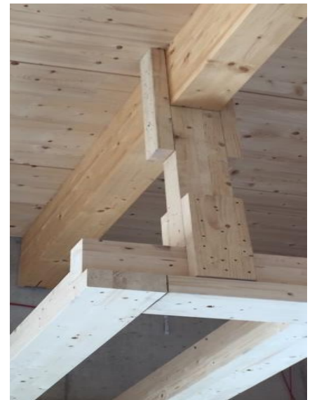
Detail Holzkonstruktion
