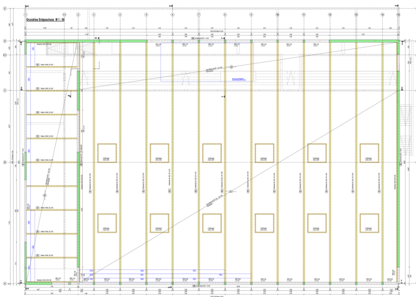
Grundriss Halle
