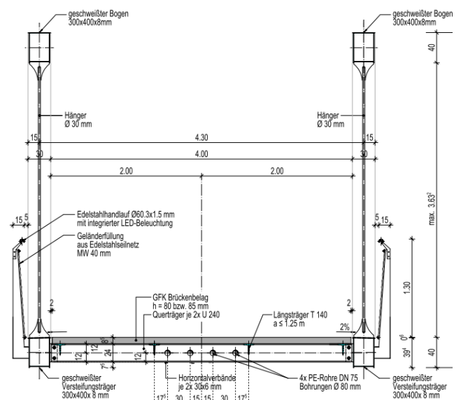
Querschnitt
