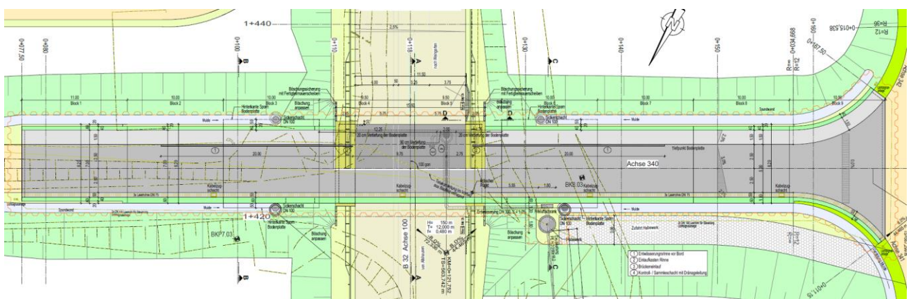
Längsschnitt und Grundriss BW 3
