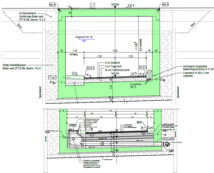
Querschnitt und Entwässerungsdetail BW 3
