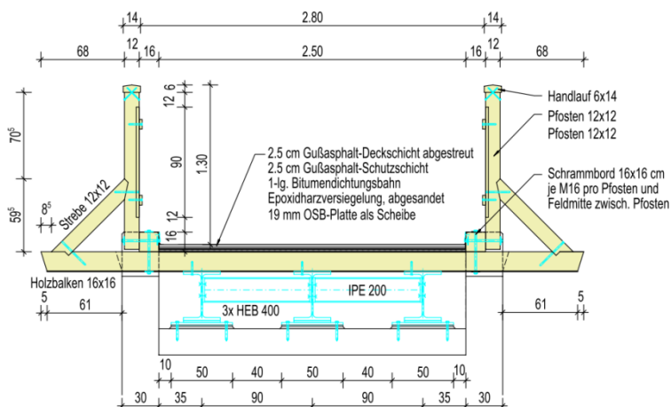
Querschnitt
