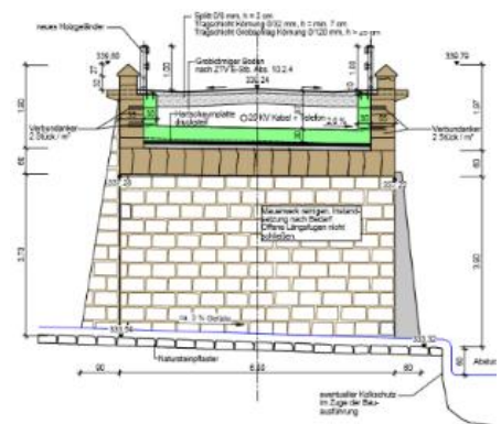
Querschnitt BW 1
