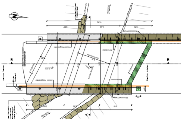
Grundriss BW 13
