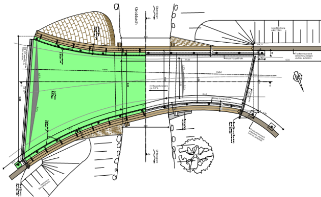
Grundriss BW 1
