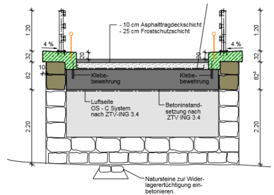
Querschnitt BW 13
