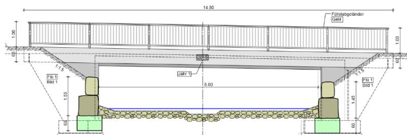
Ansicht Oberstrom
