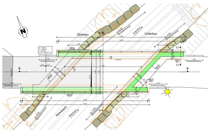
Grundriss
