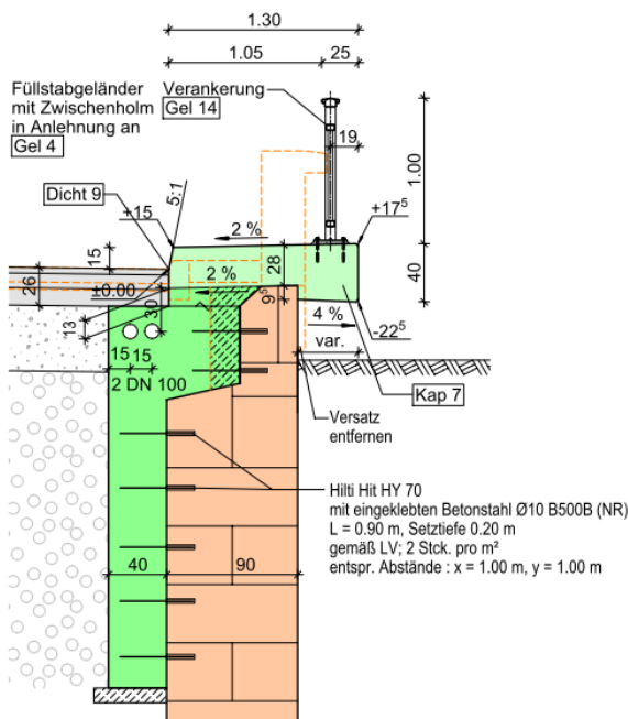
Detail hinterbetonierte Flügelwand BW 7716 558
