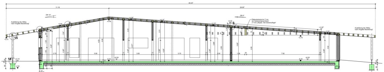
Längsschnitt Anbau
