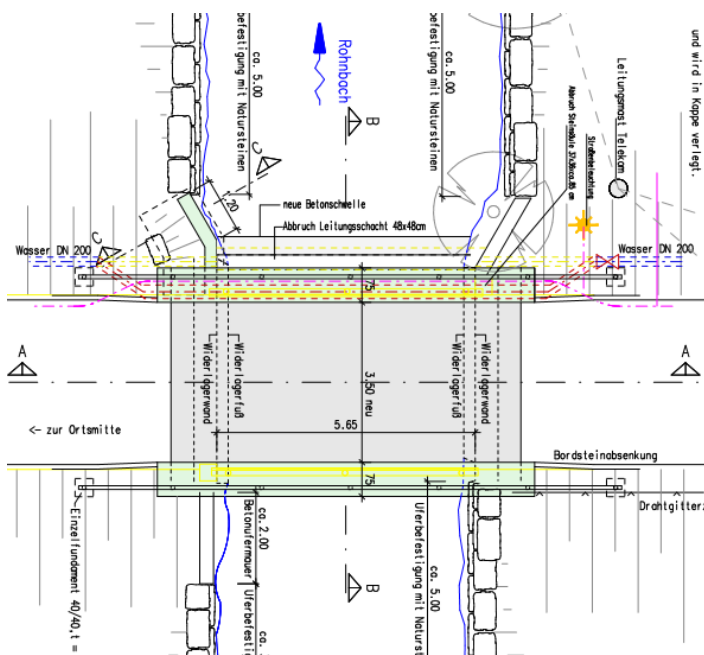
Grundriss
