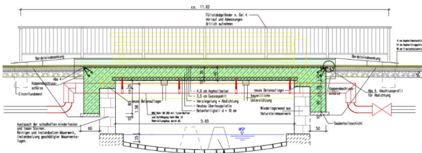
Längsschnitt
