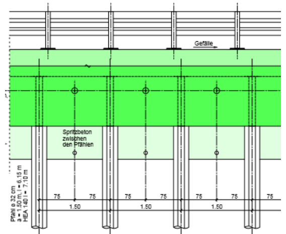
Grundriss Straße mit dauerhafter Böschungssicherung
