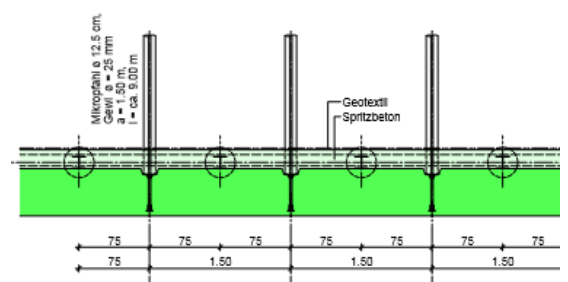
Detail Ansicht und Schnitt Stützbeton
