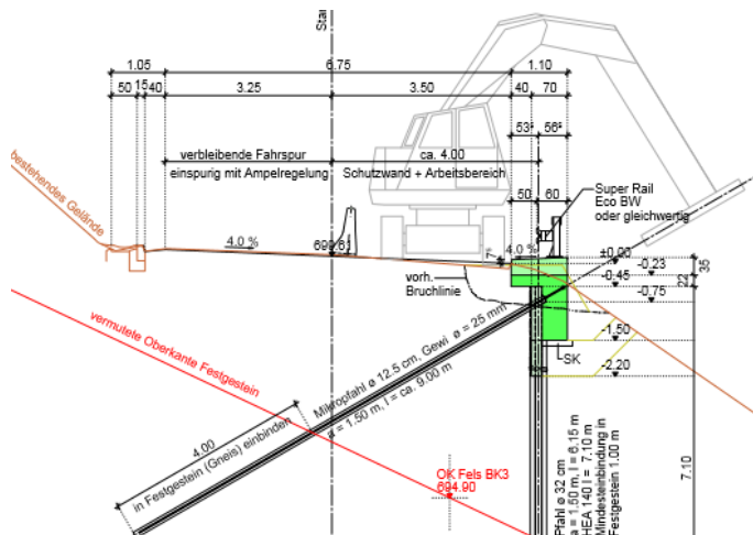
typischer Schnitt in der Bauphase
