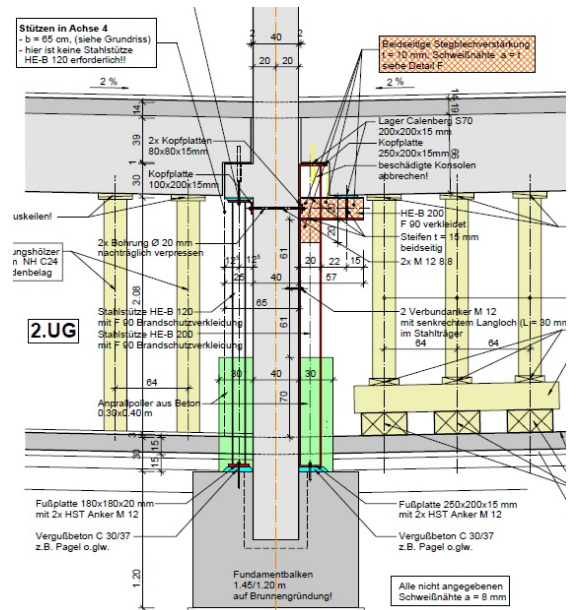
Plandetail Instandsetzung Konsole
