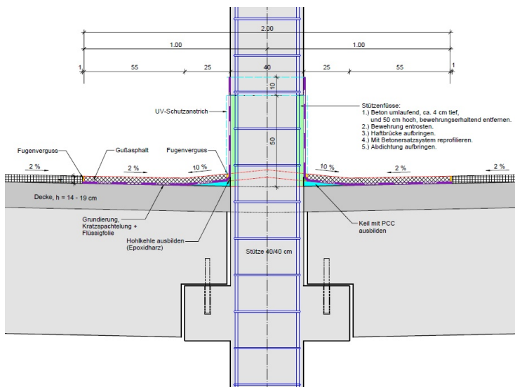
Plandetail Instandsetzung Stützenfuß
