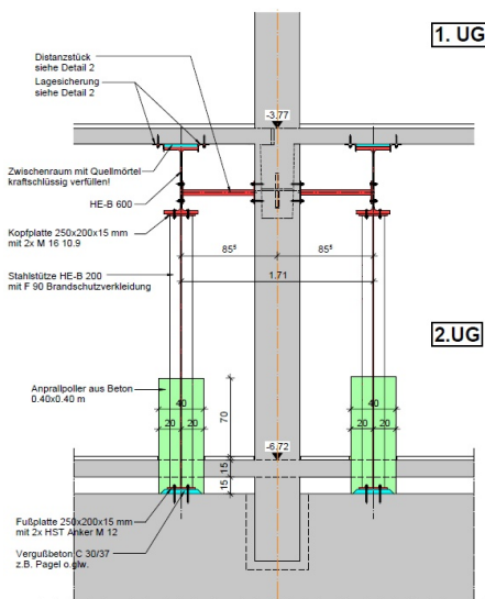
Plandetail Auflager Abfangträger
