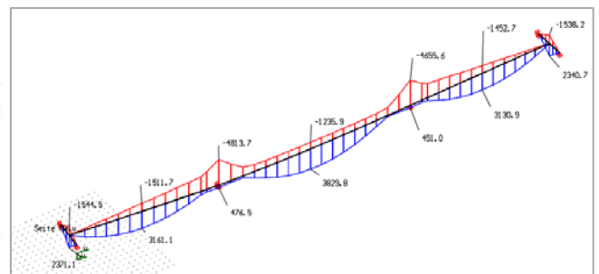
Momentenlinie Längsträger (Auszug Nachrechnung)
