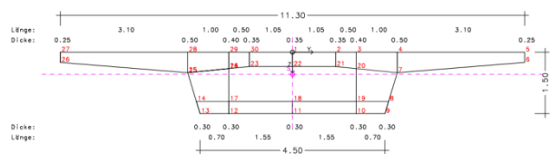
Brückenquerschnitt (Auszug Bewehrungsplan bzw. Nachrechnung der Querschnittsausnutzung)
