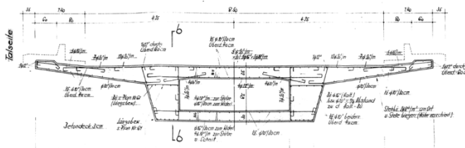
Brückenquerschnitt (Auszug Bewehrungsplan bzw. Nachrechnung der Querschnittsausnutzung)
