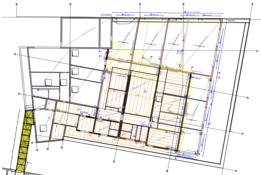
Grundriss Aufstockung und Verbindungssteg (links)
