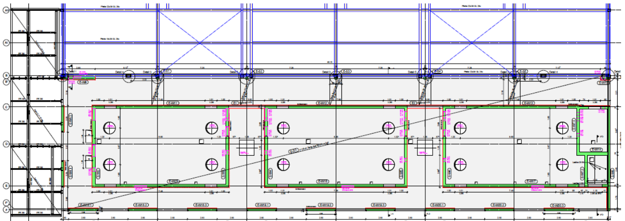
Teilgrundriss Nebentrakt und Halle
