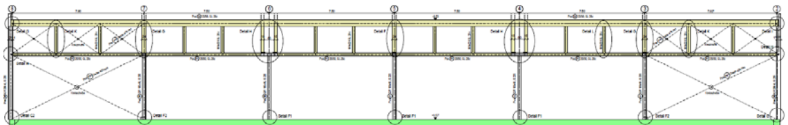
Schnitt Sporthalle
