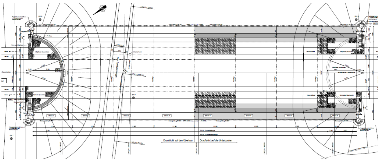
Grundriss
