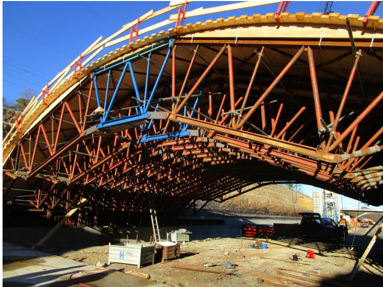
Traggerüst im Bauzustand
