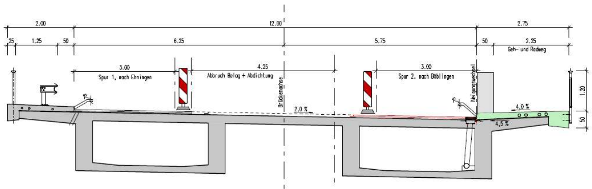
Querschnitt mit Verkehrsführung im 2. Bauabschnitt
