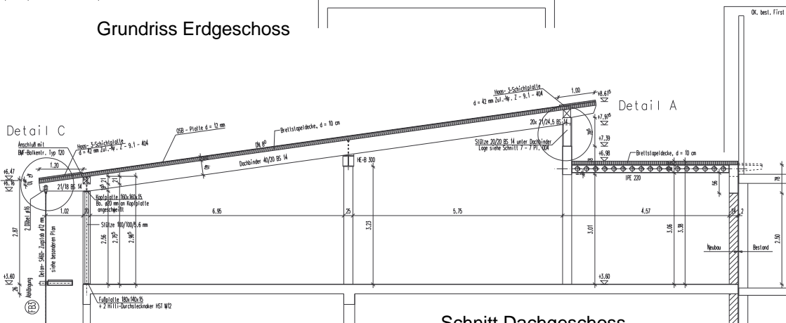
Schnitt Dachgeschoss
