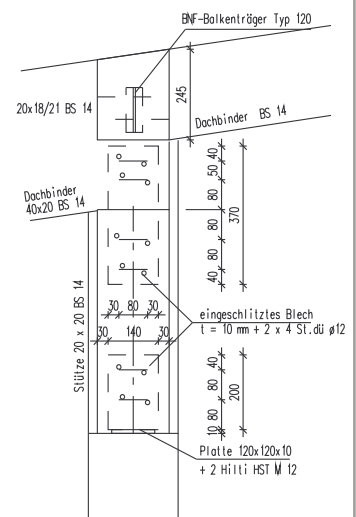
Dachdetail
