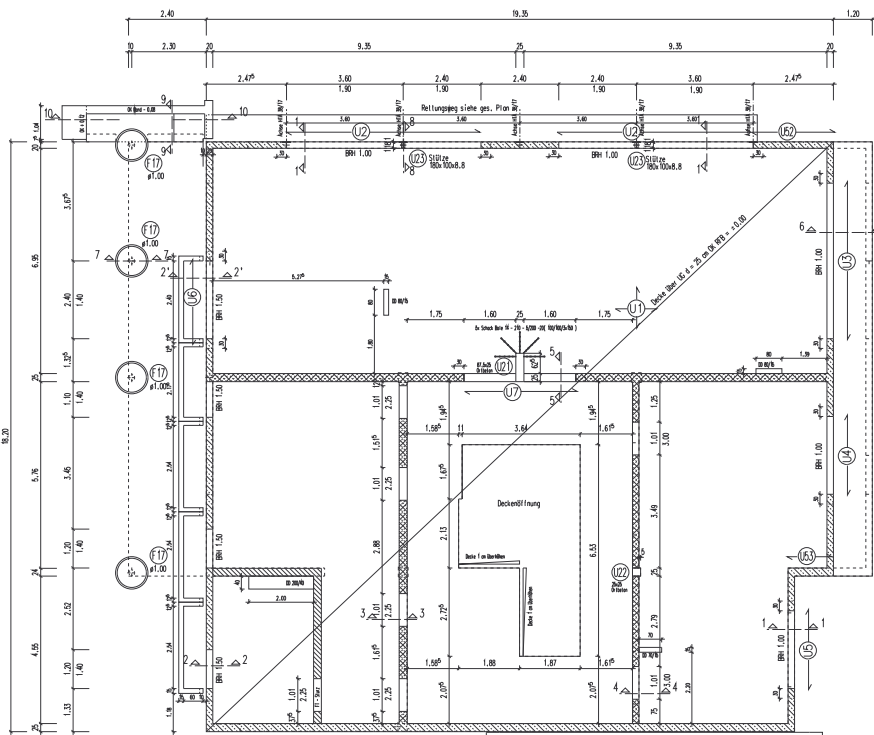
Grundriss Erdgeschoss
