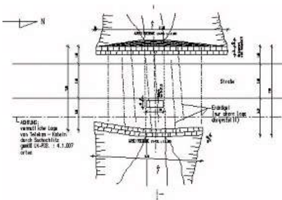
Draufsicht
