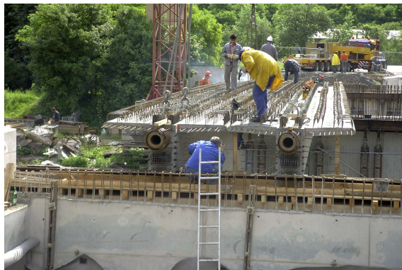
Einbau Fertigteile
