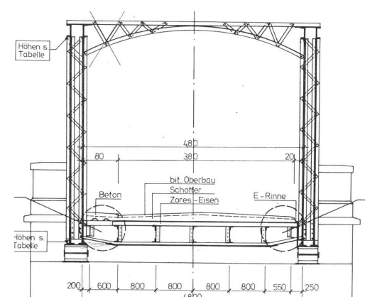
Querschnitt (Brückenbreite ca. 4.80 m)
