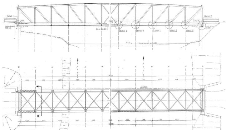
Ansicht und Grundriss (Brückenlänge 46.20 m)
