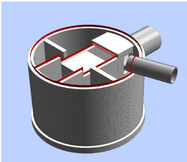
3d-Darstellung der Betonierphasen Düker-Oberhaupt
