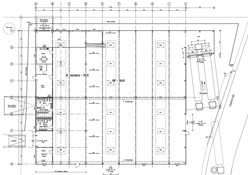
Grundriss Erdgeschoss Produktionshalle (Auszug aus Baugesuch)
