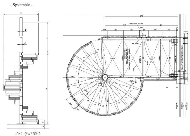
Ansicht und Grundriss Stahltreppe (Planauszüge Stahlbaufirma)
