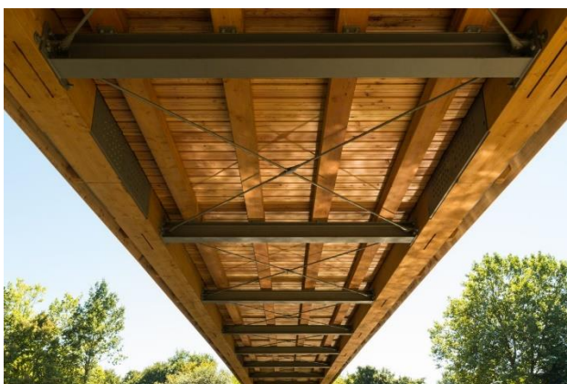
Untersicht Brücke
