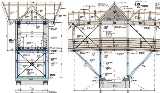
Ansicht Rahmen Mittelaugler (Auszug Plan Aufsteller und Bauausführung)
