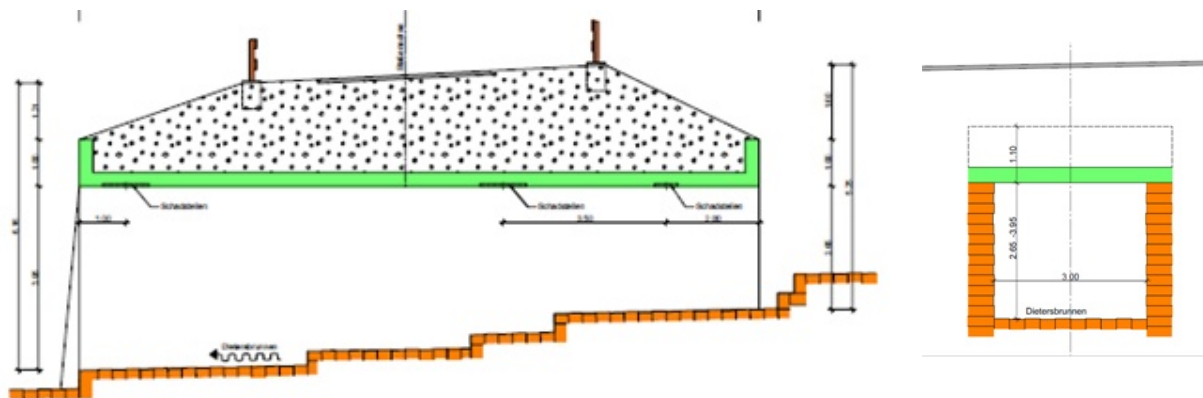
Längsschnitt und Querschnitt Dietersbrunnenbrücke
