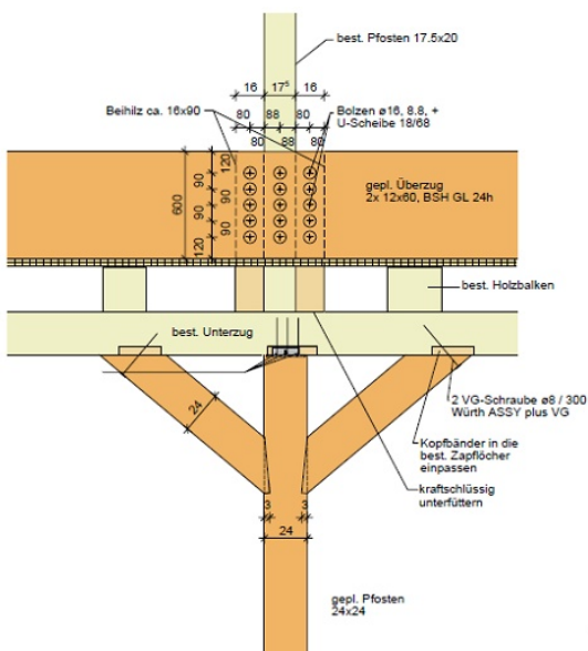
Detail Stützenkopf mit Überzug
