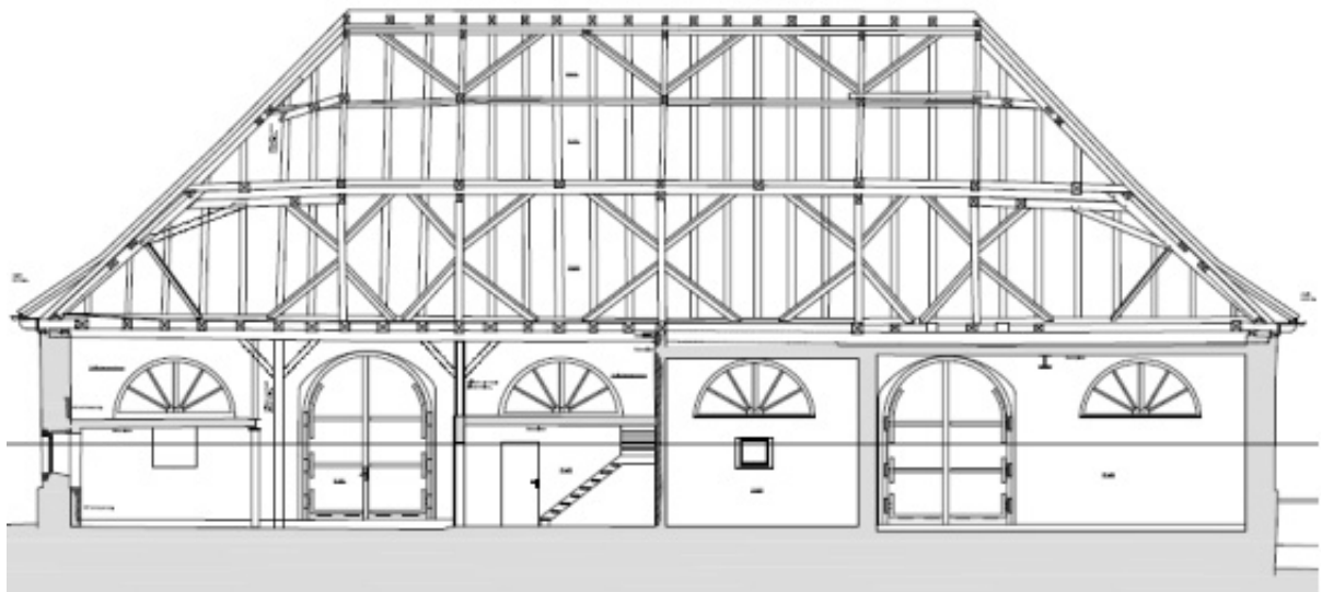
Außenansicht Bestandsplan
